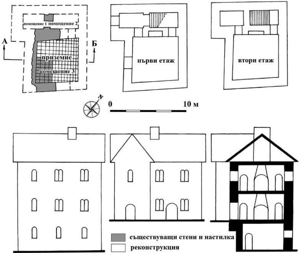
Обр. 12. Сграда № 2 под североизточния ъгъл на Царския дворец (план на приземие, първи и втори етаж; силуети на източна и западна фасади; напречен разрез) – реконструкция Е. Дерменджиев.
