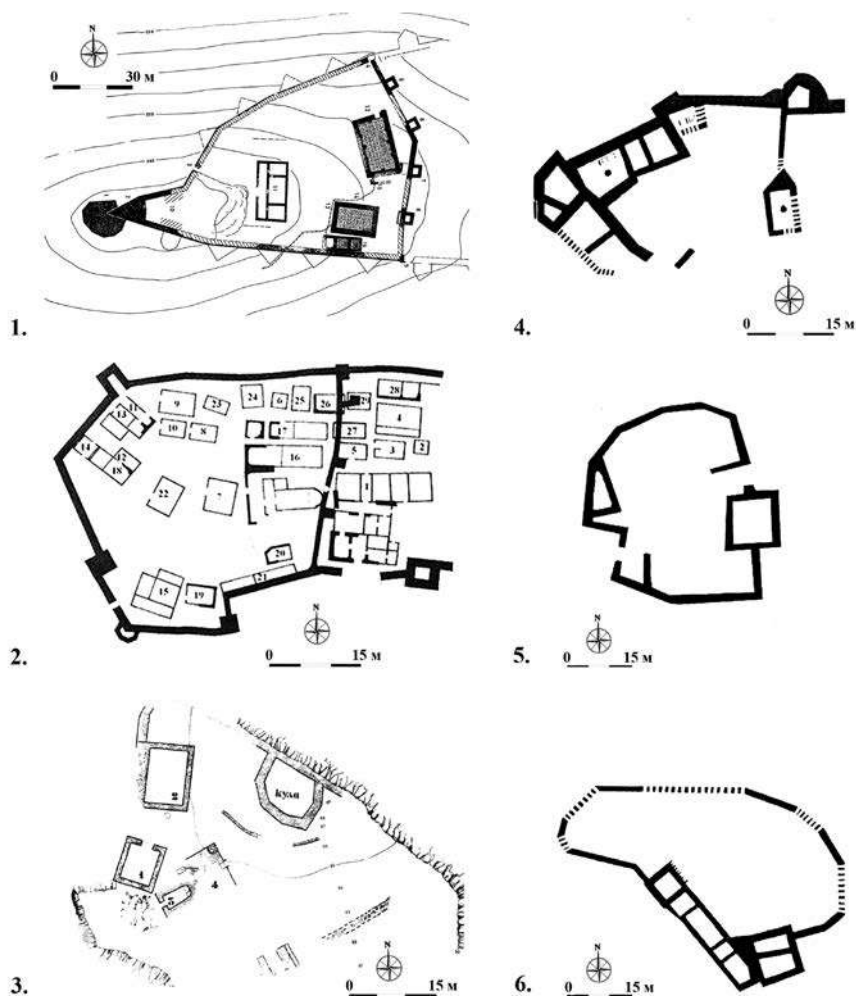
Обр. 6. Планове на малки крепости от XII–XIII в. във Византия.
