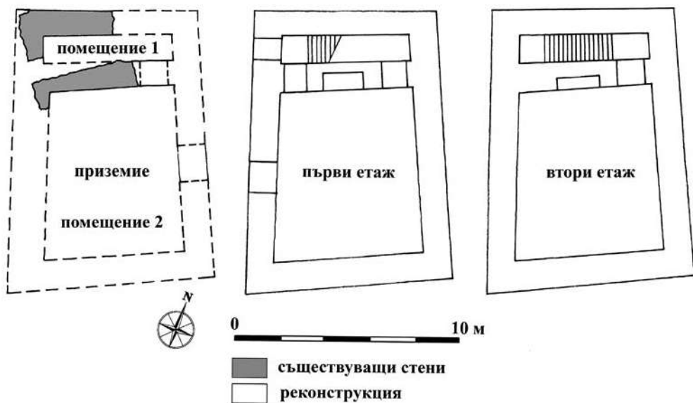
Обр. 10. Сграда №1 под североизточния ъгъл на Царския дворец (план на приземие, първи и втори етаж) – реконструкция Е. Дерменджиев.
