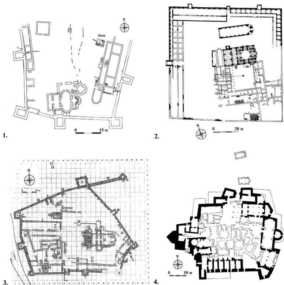
Обр. 4. Планове на укрепени манастири във Византия от XI–XII в. 1. Манастир „Св. Йоан Продром“ и епископска резиденция край Кърджали (по Н. Овчаров и Д. Хаджиева). 2. Манастирът Дафни край Атина (по P. Lazarides). 3. Манастир Зигу в Атон (по I. Papaggelos). 4. Манастир „Св. Йоан Богослов“ на остров Патмос (по X. Μπούρας).
