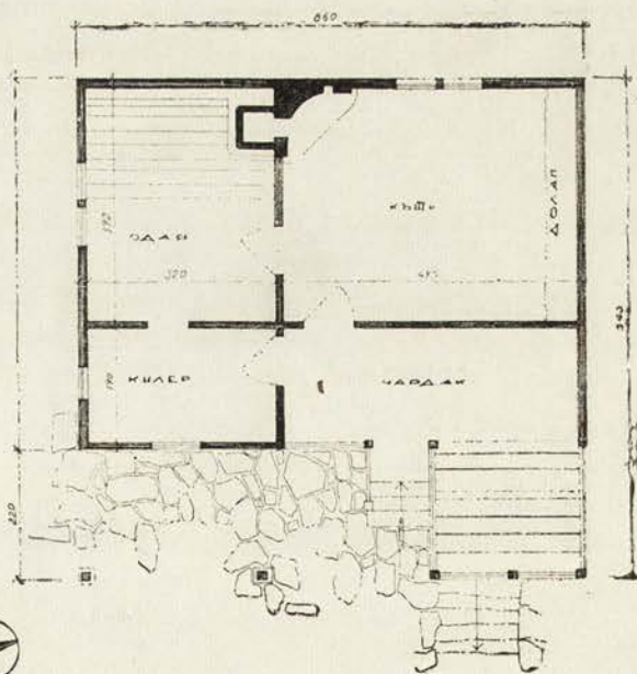
Обр. 1. Стара лясковска къща (178—г.) — разпределение
