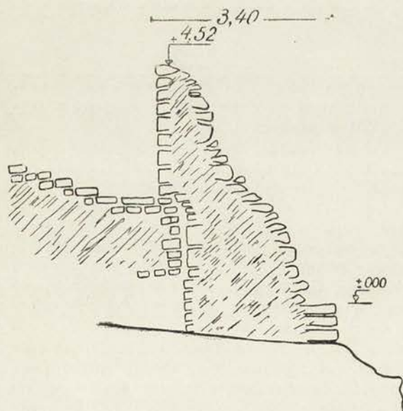
Обр. 10. Напречен разрез на крепостната стена
