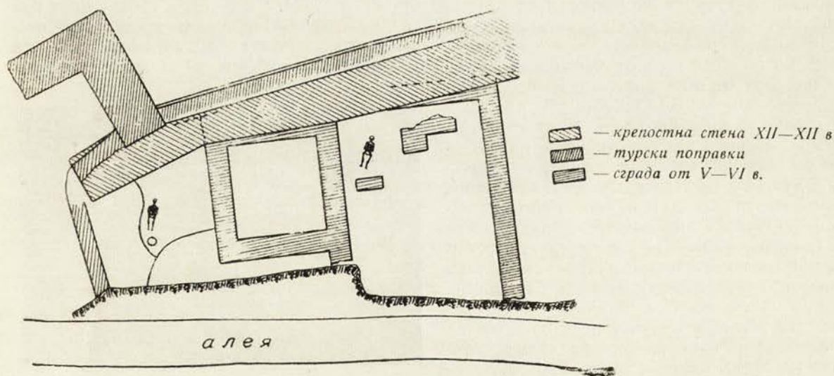
Обр. 12. Общ план на разкритата крепостна стена и сградата към нея (М 1:100)
