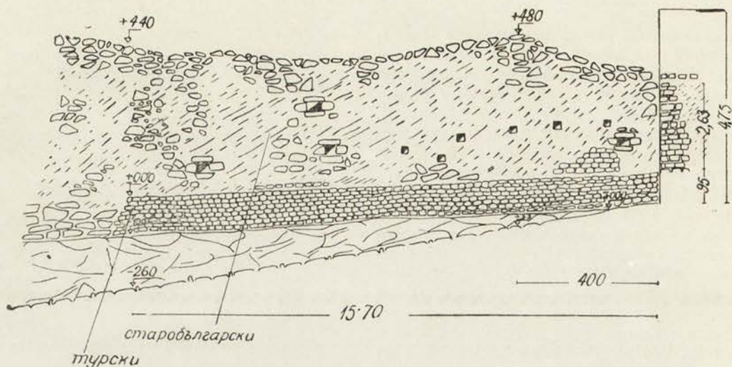
Обр. 9. Крепостната стена, гледана от външната страна
