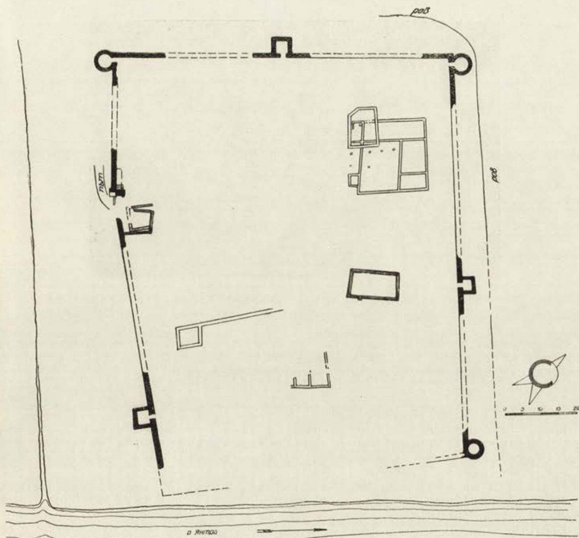
Обр. 2. Общ план на Дискодуратера
