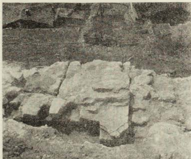
Обр. 17. Южният устой на двукрилата врата от VI в. Abb. 17. Der südliche Pfeiler der Flügeltür aus dem VI Jahrh.
