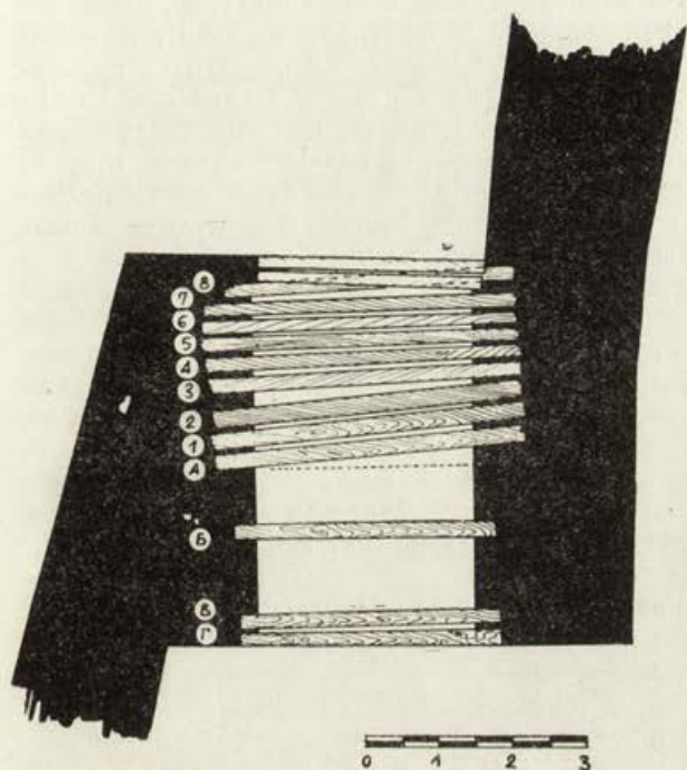
Обр. 9. Хоризонтален разрез на гредоредата на Малката порта
