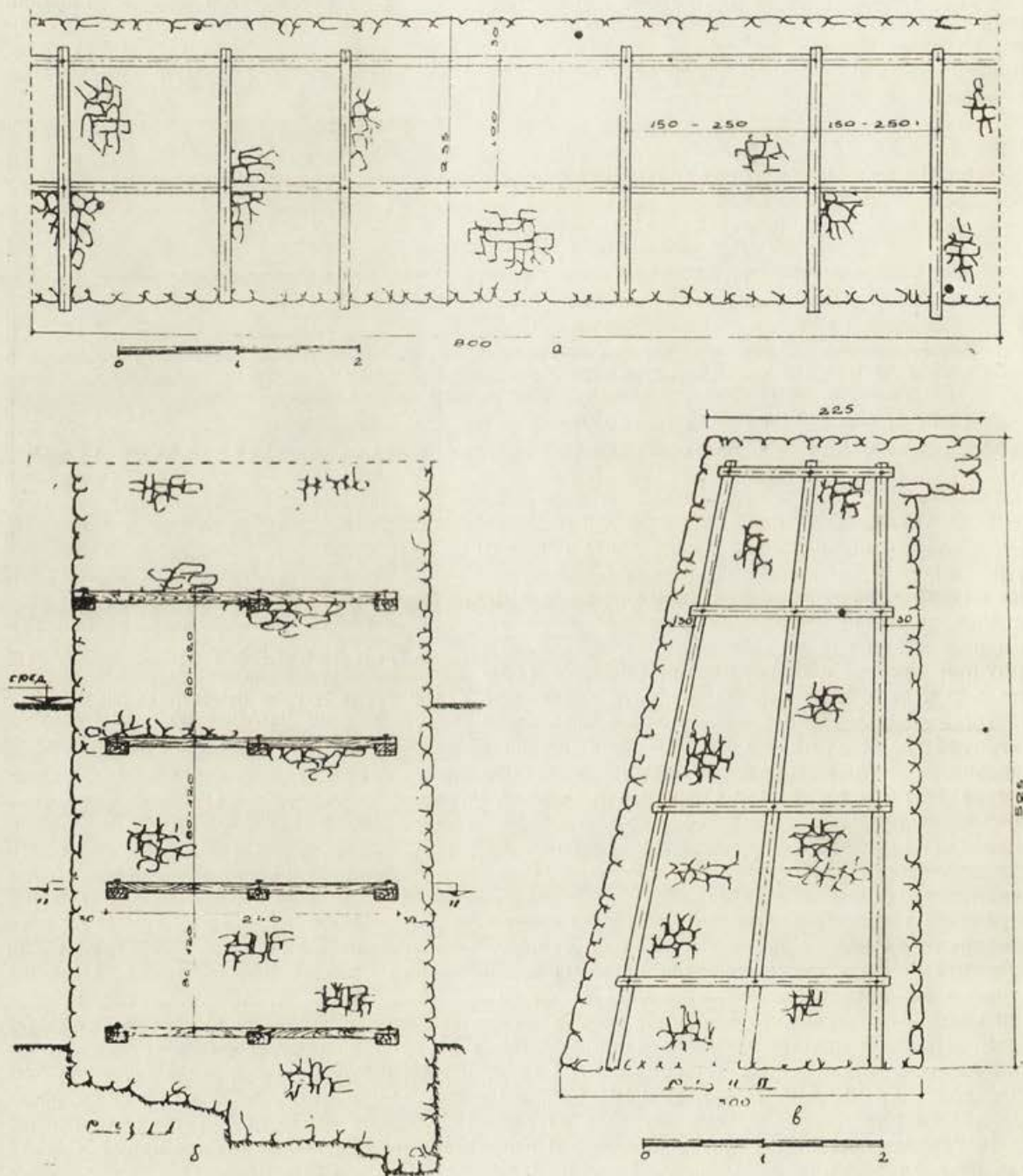
Обр. 8. Дървени скари — сантрачи — в крепостните стени и порти Abb. 8. Holzroste — santratschi — in den Festungsmauern und in den Toren
