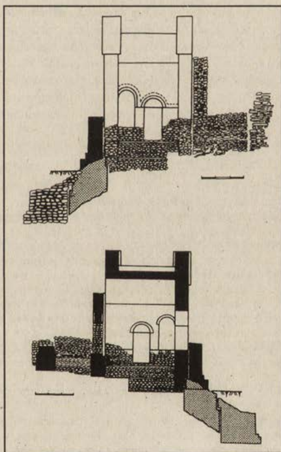
Обр. VI. Южна фасада и южна вътрешна стена на Екзонартекса - реконструкция. (Е. Дерменджиев)
