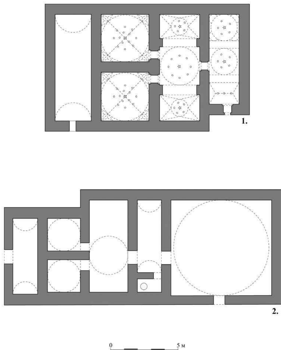
Обр. 2. Хамами с правоъгълна централна част, два айвана и два халвета в Нова Загора и Пловдив. 1. Али паша хамам в Нова Загора (по М. Кийл); 2. Баня „Марица“ в Пловдив (по М. Харбова).
