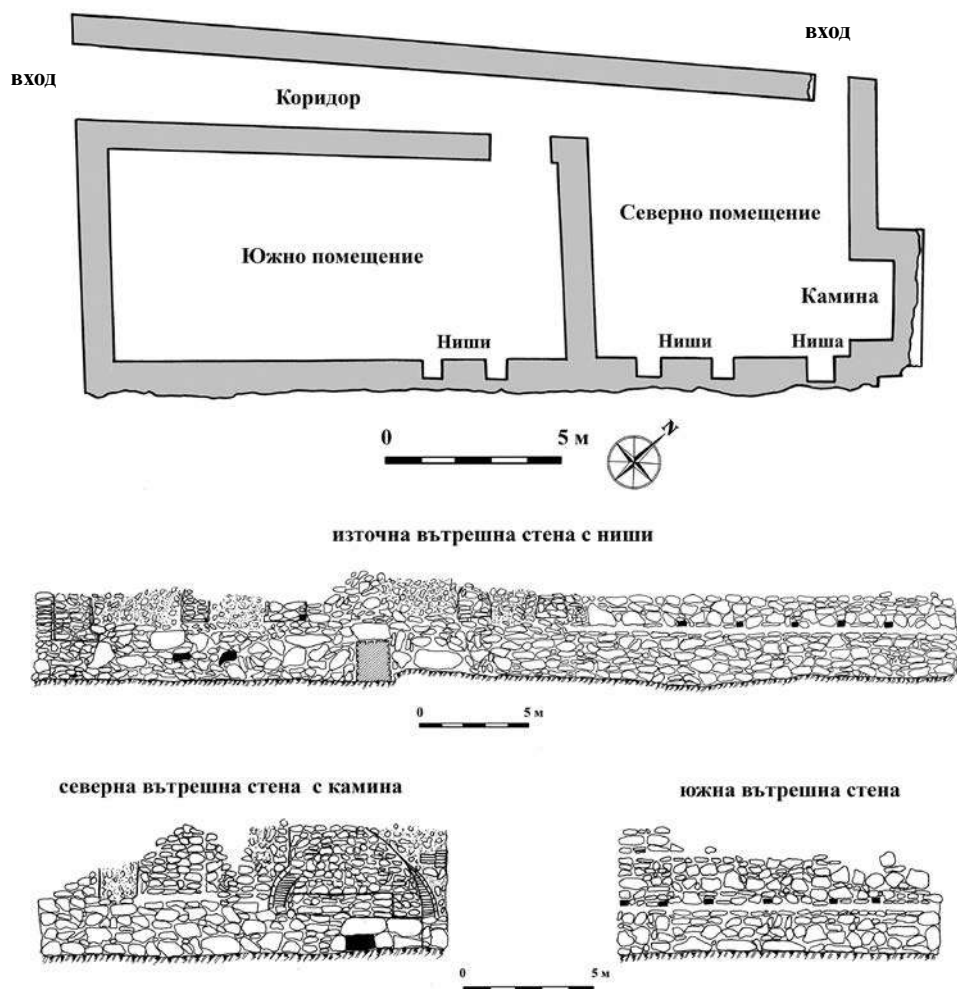
Обр. 6. План и изгледи на вътрешните стени на Сградата при Северозападната порта в цитаделата на хълма Царевец (по П. Славчев).
