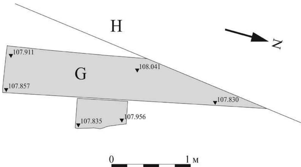
Обр. 15. План на дясната страница от акведукта: G – страница; H – стена на рибарник (чертеж К. Чакъров).
