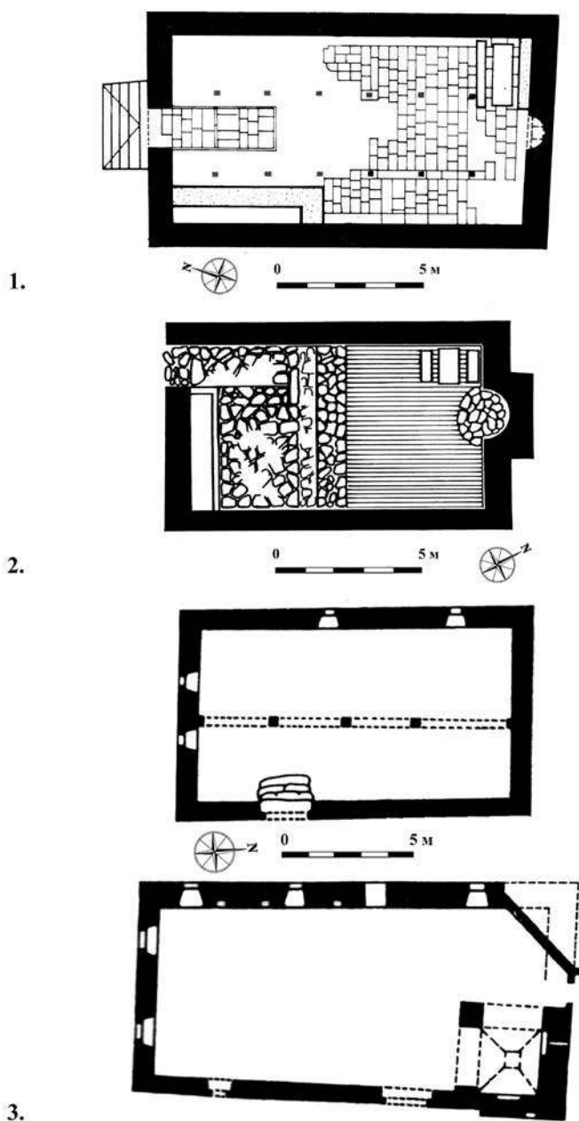
Обр. 11. Планове на средновековни странноприемници от XIII – XIV в. в България (по Н. Тулешков). 1. Червен; 2. Калиакра; 3. Метох „Орлица“ на Рилски манастир – приземие и горен етаж.
