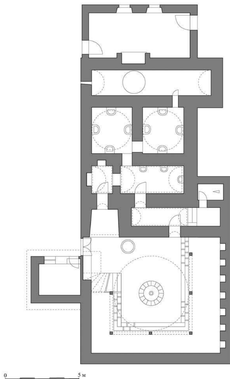
Обр. 6. Хамам с правоъгълна централна част и два халвета в Карлово (по Д. Попов).
