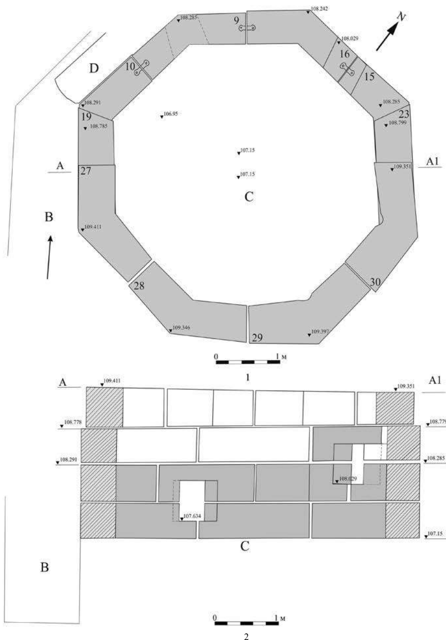
Обр. 6. Общ план и напречен разрез на каптажа (чертежи К. Чакъров). 1. Общ план: В – подземна скална галерия; С – каптаж; D – зид между каптажа и галерията; 2. Напречен разрез. Fig. 6. General plan and Cross-section of the Water Catchment (drawings K. Chakarov). 1. General plan: B – Underground Cut in the Rock Gallery; C – Water-catchment; D – Wall between the Water-catchment and the Gallery; 2. Cross-section.
