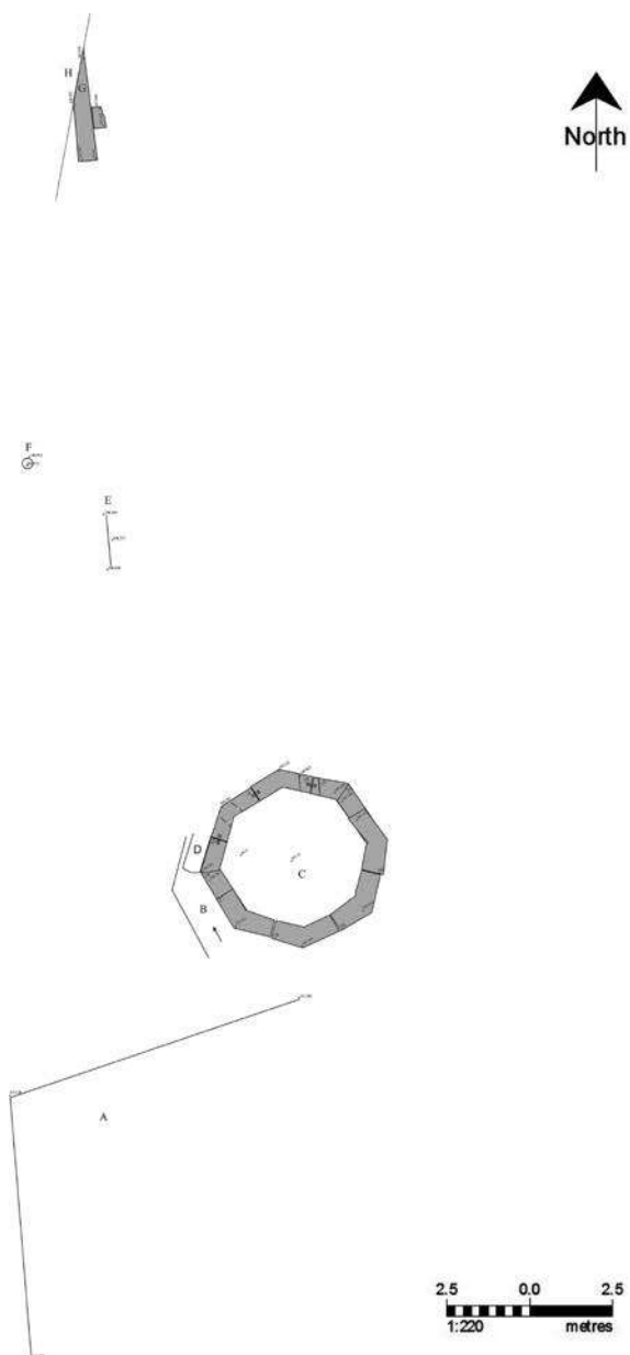
Обр. 12. План на каптажа и структурите около него: A – стара мелница; B – скална галерия; C – каптаж; D – зид в галерията; E – скално засичане; F – дупка в скалата; G – страница от акведукта; H – съвременен рибарник (чертеж К. Чакъров).
