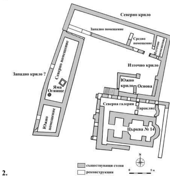
Обр. 3. План на Комплекса до църква № 14 в цитаделата на хълма Царевец (по Х. Нурков и А. Писарев).
