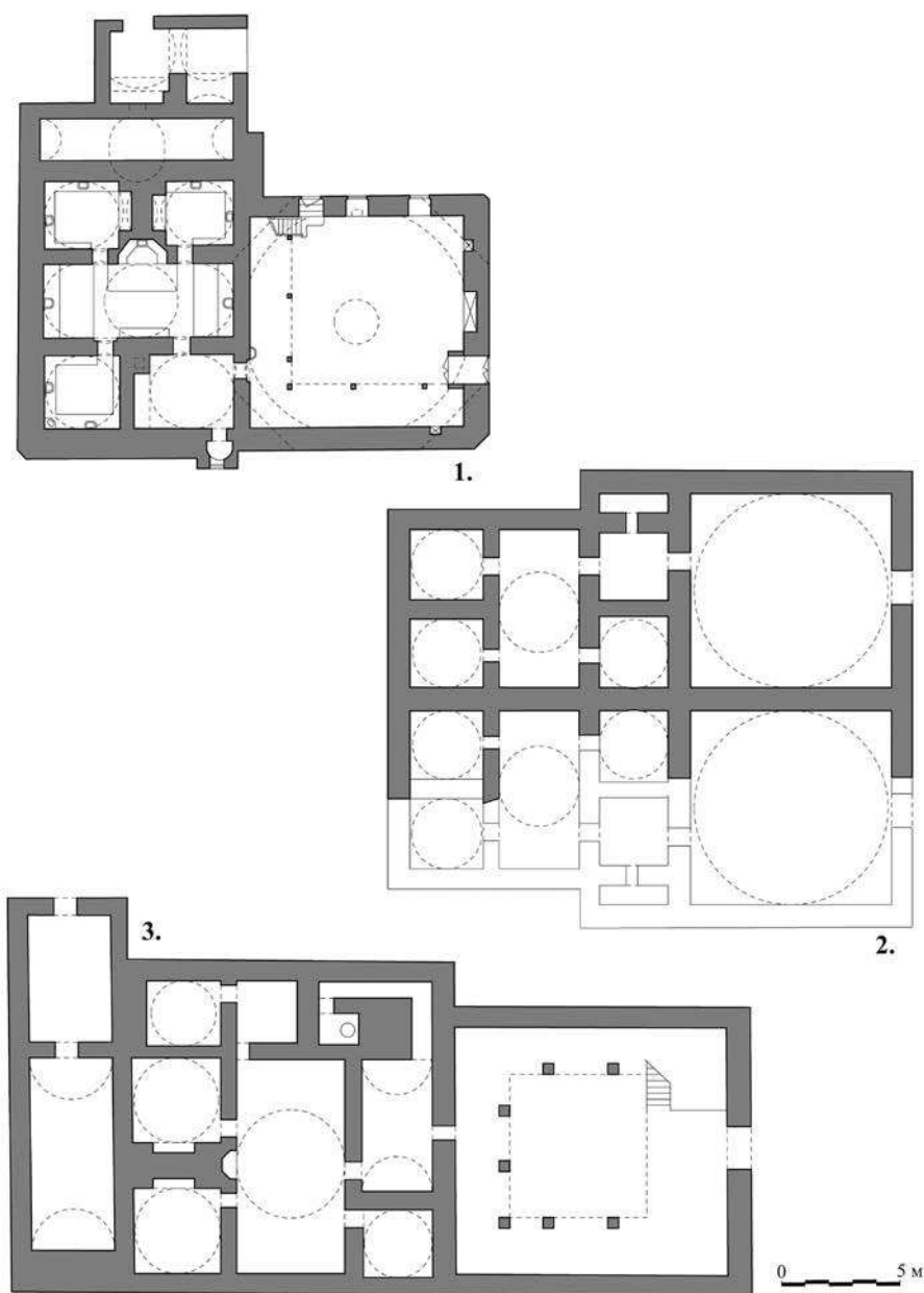
Обр. 3. Хамами с правоъгълна централна част, два айвана и три халвета в Ловеч, Видин и Пловдив. 1. Дели хамам в Ловеч (по К. Калев); 2. Чифте хамам във Видин (по М. Харбова); 3. Орта Мезар хамам в Пловдив (по М. Харбова, с добавки на автора).
