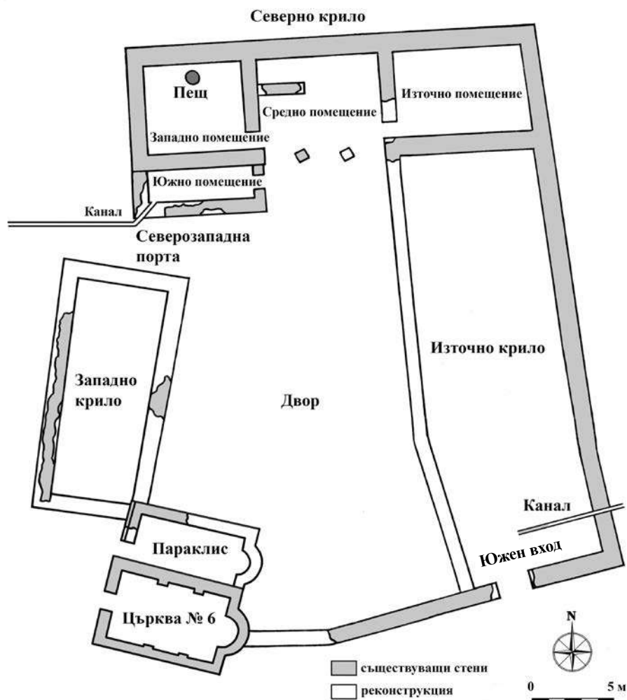
Обр. 5. План на Комплекса до Църква № 6 в цитаделата на хълма Царевец – реконструкция Е. Дерменджиев (по Я. Николова).
