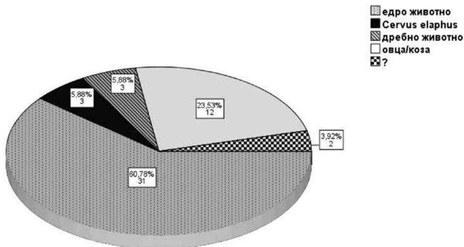
Обр. 8. Графика с разпределение на видовете животни, костите от които са използвани за изготвянето на предметите от Хотница – Извора.
