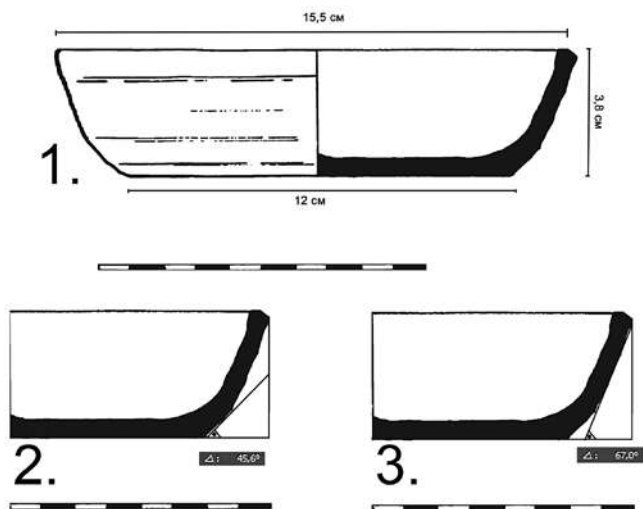
Обр. 1. Профил на паница № 1415 A/TOM – рисунки. 1. Цял профил; 2. Първи ъгъл на изкачване от дъното – детайл; 3. Втори ъгъл на източване на стените – детайл.
