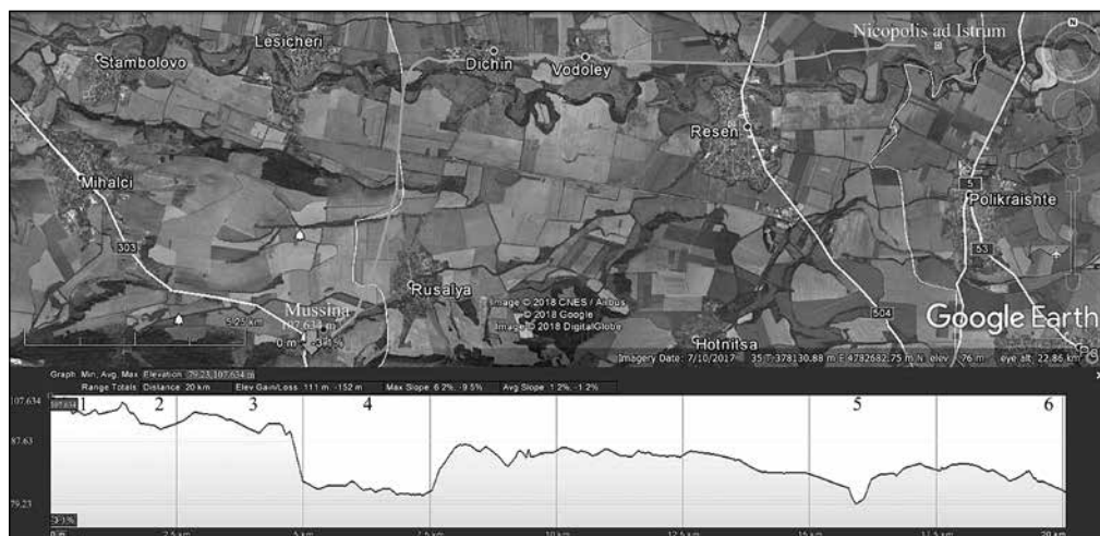
Обр. 17. Трасе на Западния акведукт на Никополис ад Иструм и разрез на терена с ардаки: 1 – над река Пещерска (?); 2 – над река Негованка; 3 – над Бабино/Кору дере; 4 – над река Росица; 5 – над река Барата; 6 – пред castellum aquae (Google Earth; К. Чакъров).
