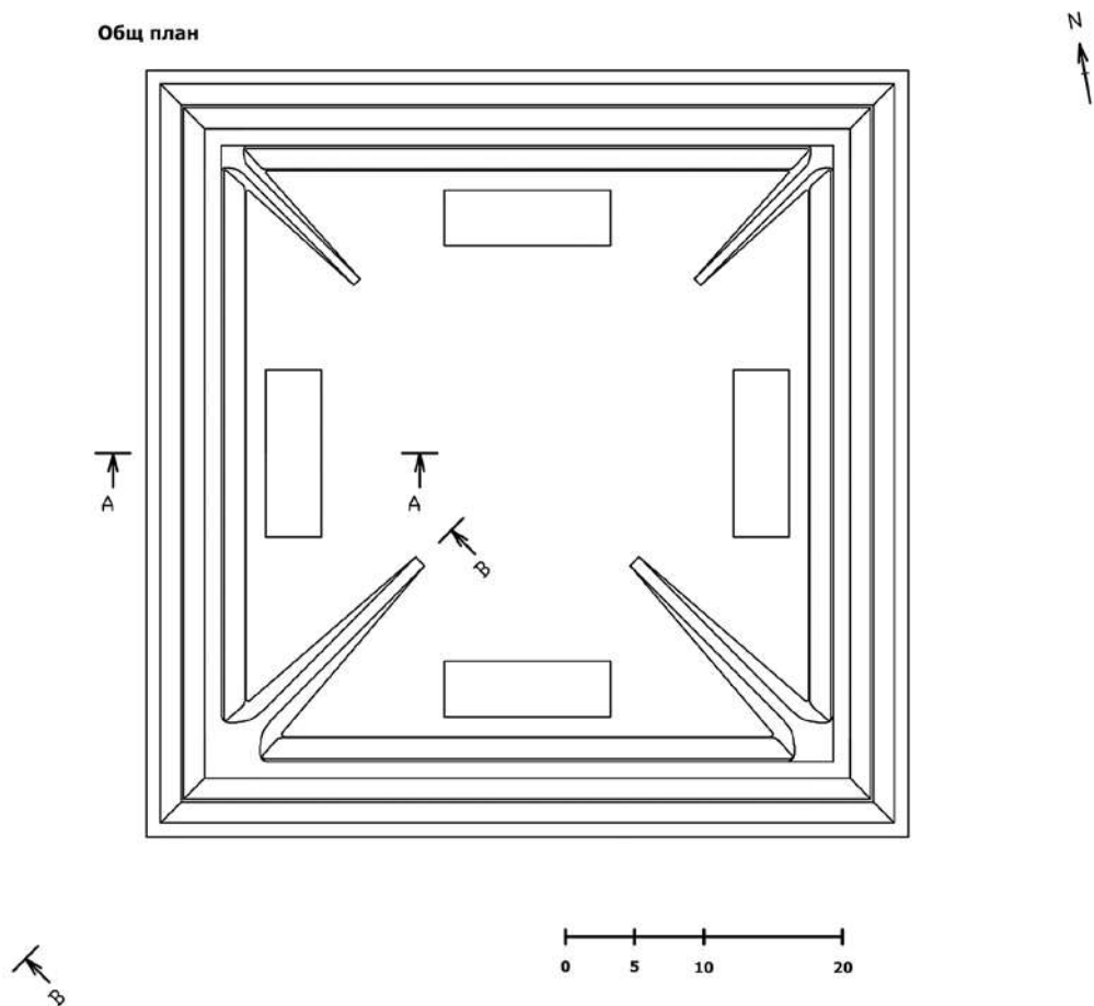
Обр. 3. Приблизителен план и разреди на табията на хълма Гарга баир. Fig. 3. Approximate plan and sections of the tabbion the hill of Garga Bair.
