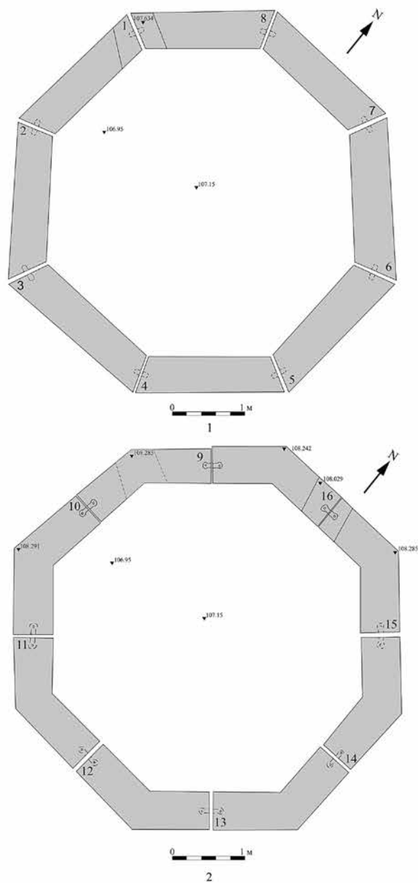
Обр. 7. План на каптажа (чертеж К. Чакъров).
