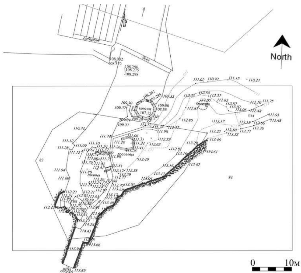
Обр. 1. Геодезическа снимка на района около каптажа и Мусинската пещера. Fig. 1. Geodesy of the Area around the Water-catchment and the Mussinska Cave.
