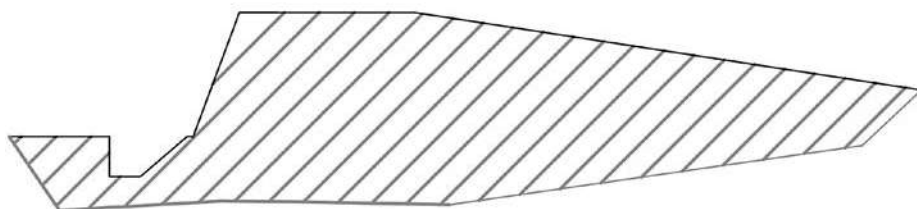
Напречен разрез на югозападния апарел (В-В)
