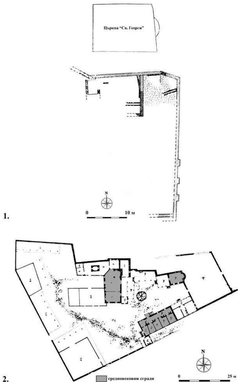
Обр. 12. Планове на средновековни странноприеминици от XI – XIV в. в България (по Н. Тулешков). 1. Метох „Св. Георги“ на Бачковски манастир 2. Метох „Орлица“ на Рилски манастир.
