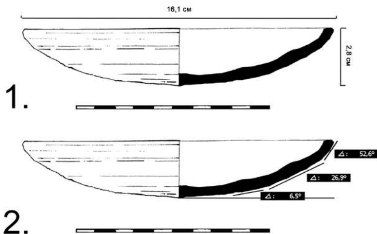
Обр. 8. Профил на паница № 1416 A/TOM – рисунки.
