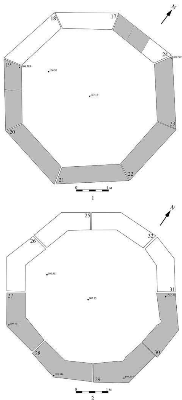
Обр. 8. План на каптажа (чертеж К. Чакъров).
